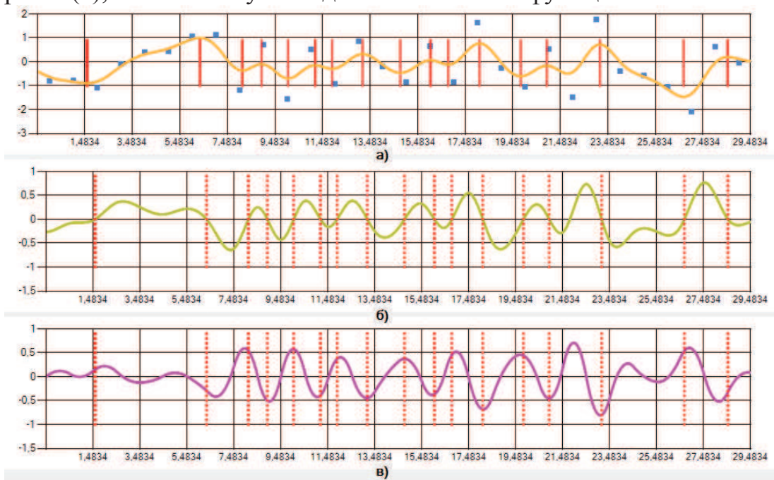
Рисунок 1 – Реалізація аналогового сигналу та згладжування його за допомогою сплайнів: а) відліки сигналу та сплайн S_{4,0}(p, t) ; б) сплайн S'_{4,0}(p, t) ; в) сплайн S''_{4,0}(p, t) .
